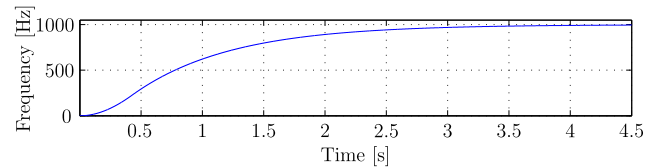
(d) Electrical frequency of the machine.
